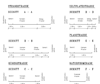
nachrichtlich: STASSENQUERSCHNITTE M: 1: 100
