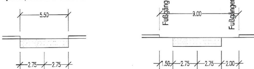
Systemquerschnitte Planstraße
