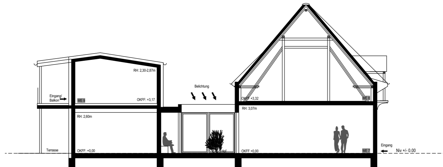
Schnitt C
