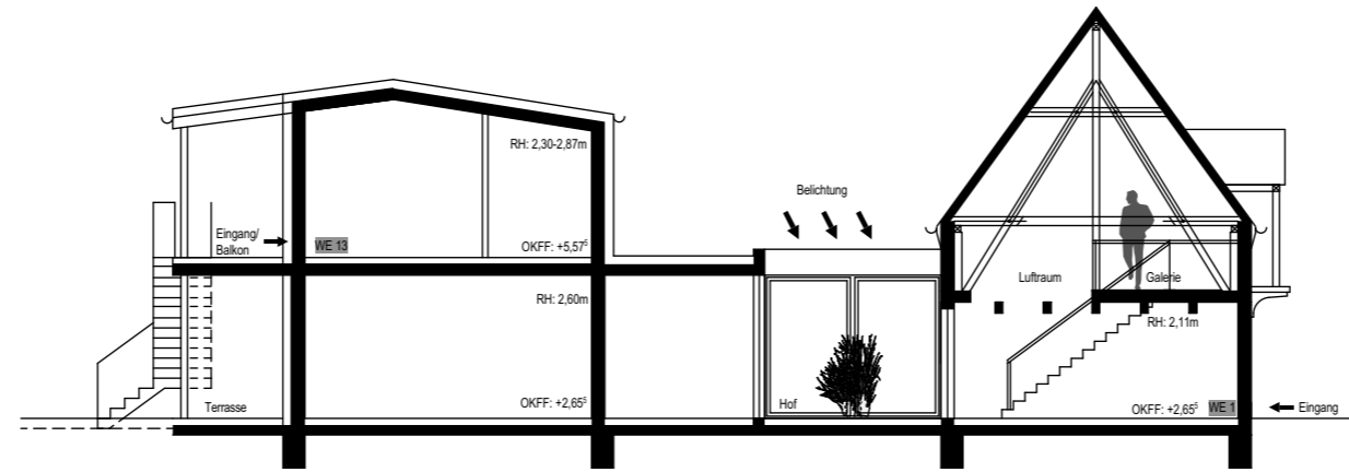
Schnitt A
