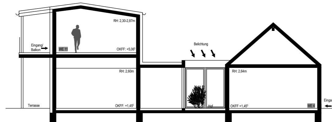
Schnitt B
