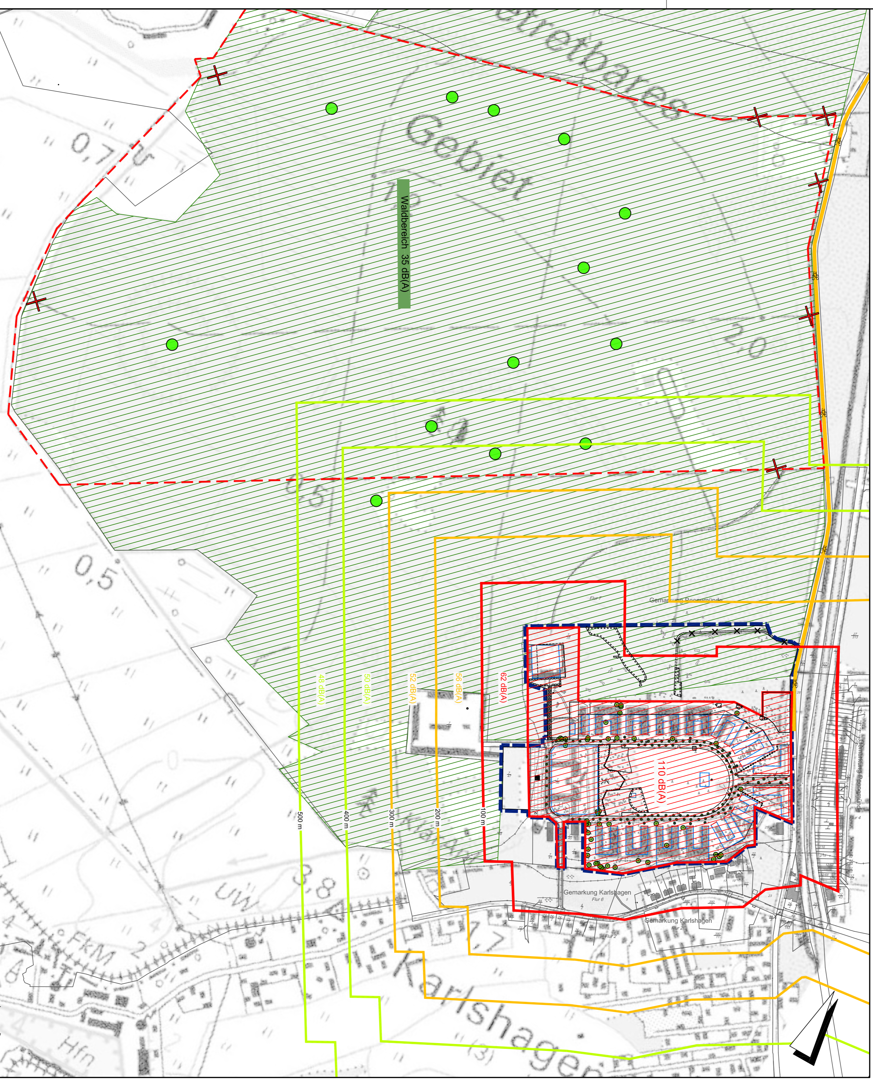
Isophonenbetrachtung für Bauphase unter Annahme von 110 dB(A) Mittelungsspiegel
